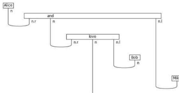
Fig. 6. Diagrama en forma normal
