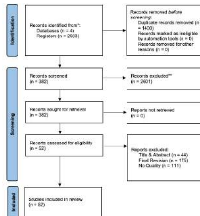
Fig. 1. Diagrama Prisma
