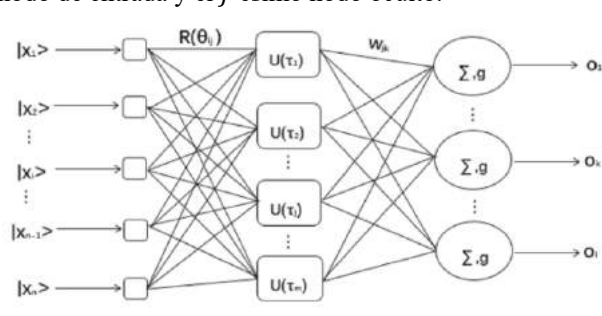
Fig. 3. Red neuronal cuántica con retropropagación
