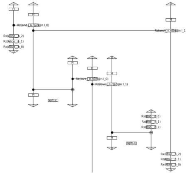
Fig. 7. Ansatz generado a partir del IQP ansatz
