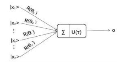
Fig. 2. Neurona cuántica
